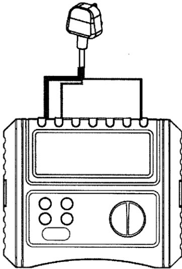
Fig. 5 Masurarea tensiunii/frecventei
