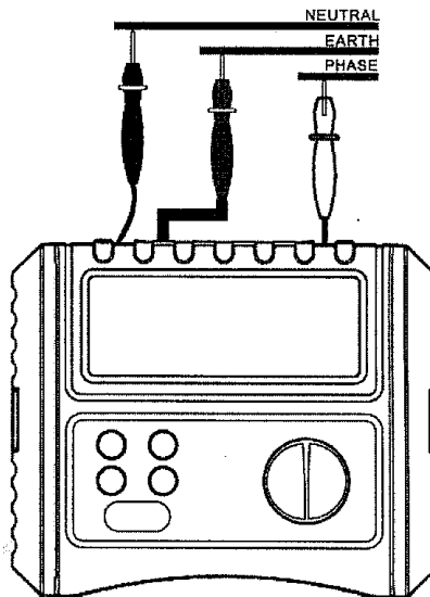
Fig. 7 Masurarea impedantei buclei
