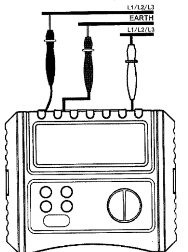
Fig. 8 Masurarea impedantei interne intre faze
